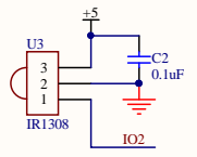
一体化红外接头
