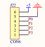
额外扩展口（使用PCF8574后四个口）
